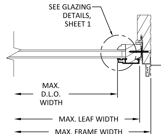
H HORIZONTAL SECTION 6 TYP. JAMB
